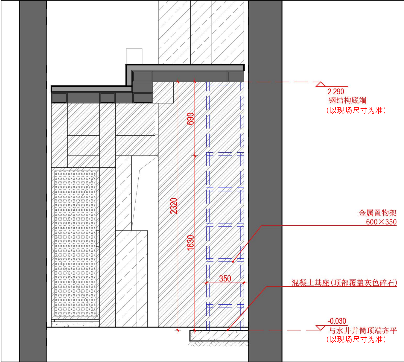
剖面图
