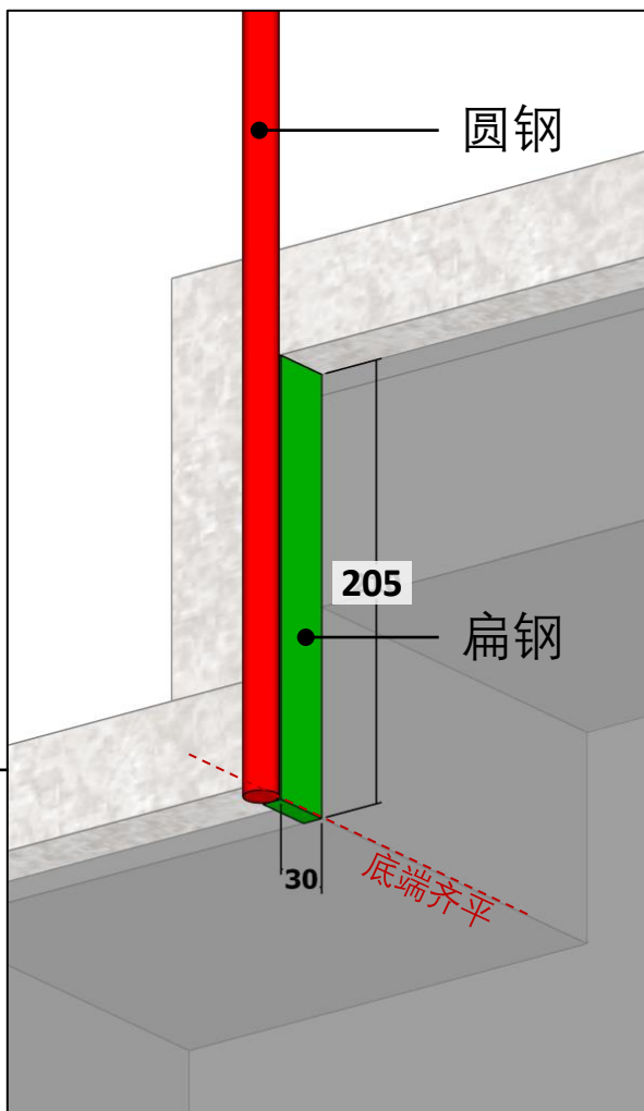
底部固定点做法 (焊接处需打磨, 使表面平整美观)
