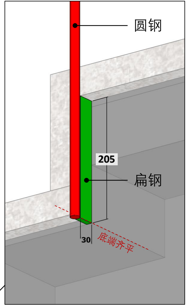
底部固定点做法 (焊接处需打磨, 使表面平整美观)
