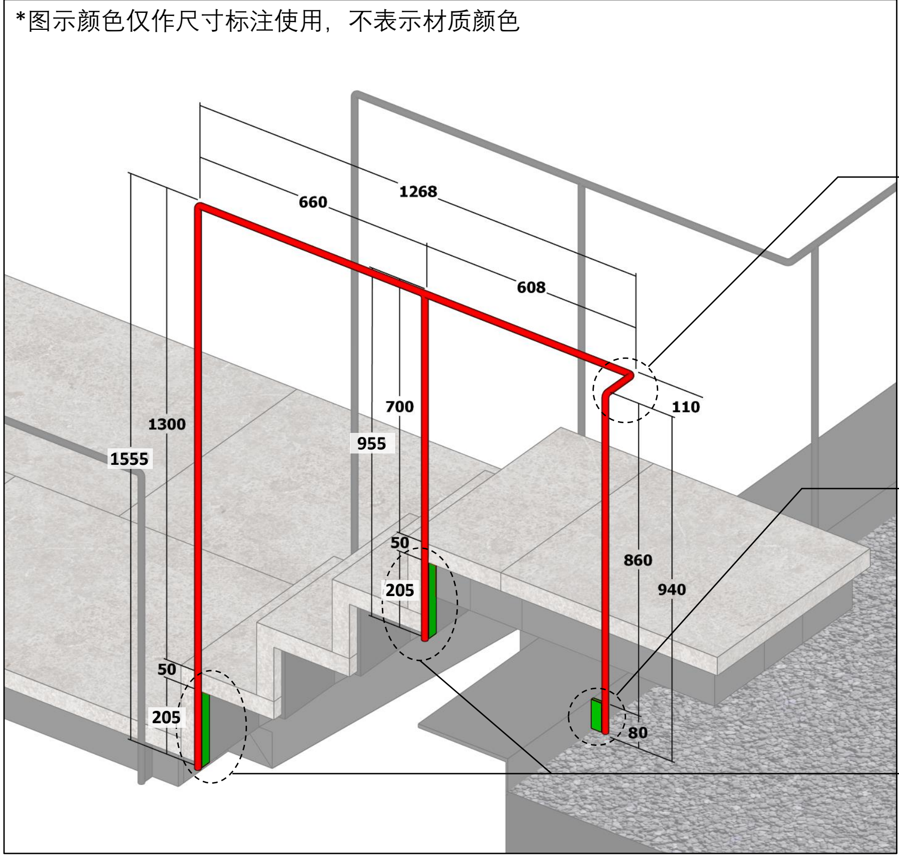
底部固定点做法 (焊接处需打磨, 使表面平整美观)
