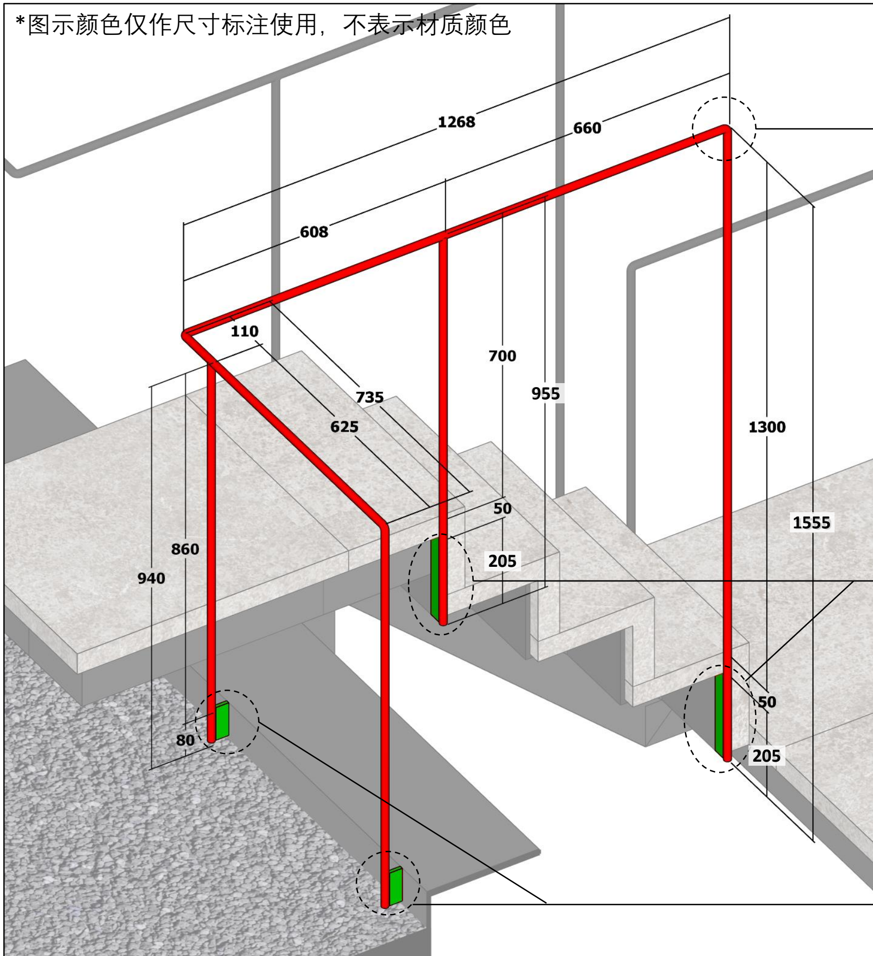
底部固定点做法 (焊接处需打磨, 使表面平整美观)
