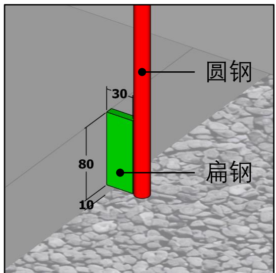
底部固定点做法 (焊接处需打磨, 使表面平整美观)
